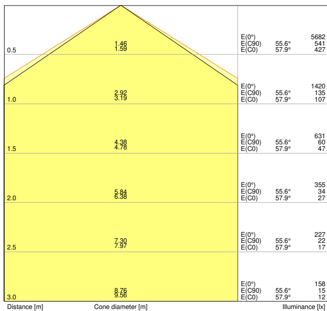
PL CMFT 1200 P 33W 830 DALIVR
