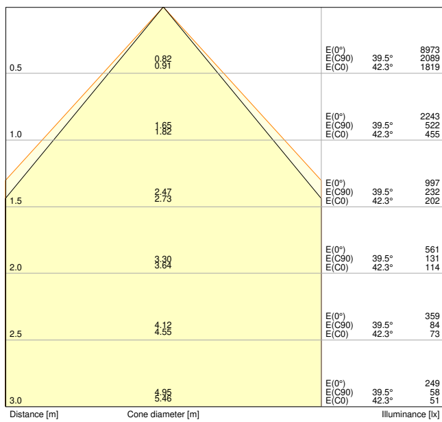
PL CMFT 600 ZB P 33W 830 U19 LEDV
