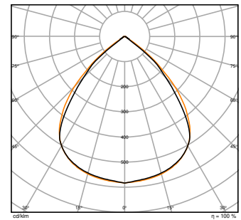
LB FLEX 1200 P 73W 840 W
