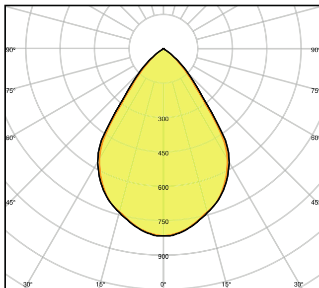
DL COMFORT DN130 13W3CCT 60DEG WT-4000K
