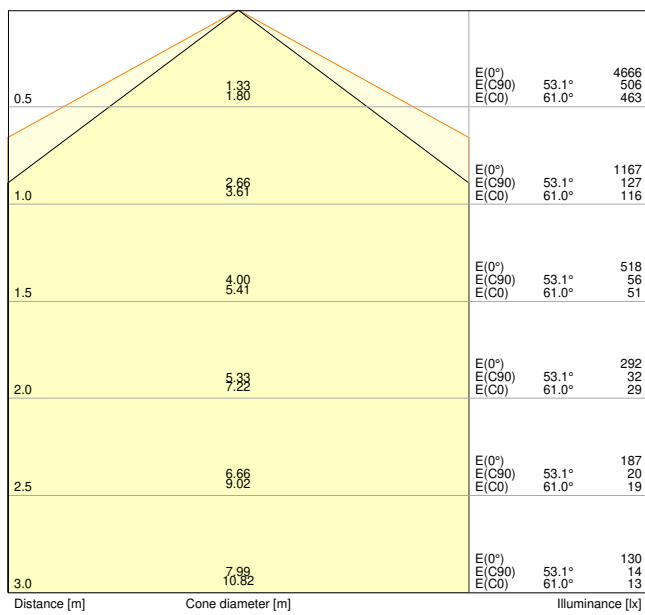
DP MAX EL 1500 S 41W 840 VW IP69 LEDV
