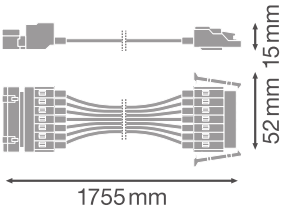
TRUSYS UNIV 1500 7P WIRE
