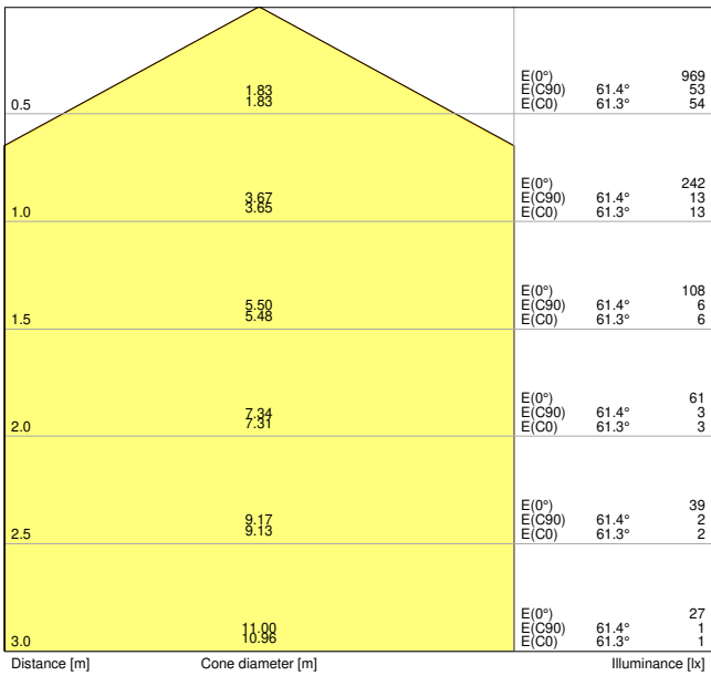
SF CIRC 250 SEN V 13W 840 IP44
