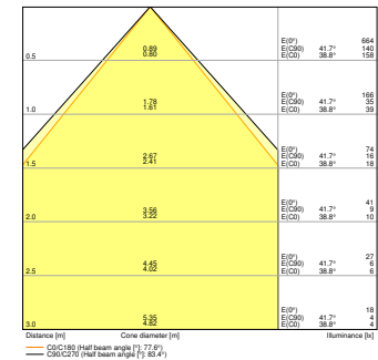
PL CMFT 600 P 33W 865 U19 DALIVR EM CONVERSION BOX
