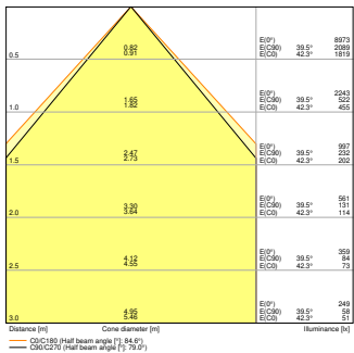
PL CMFT 600 P 33W 840 U19 DALIVR
