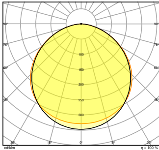
PL CMFT 1200 P 33W 840 DALIVR
