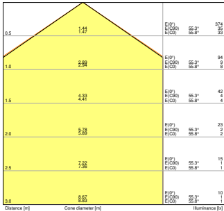
PL CMFT 1200 P 33W 840 DALIVR EM CONVERSION BOX
