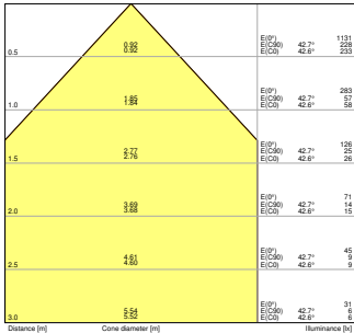
PL CMFT 1200 P 33W 840 DALIVR EM
