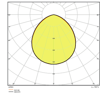
FL PFM 30W3000K SYM 100 BK
