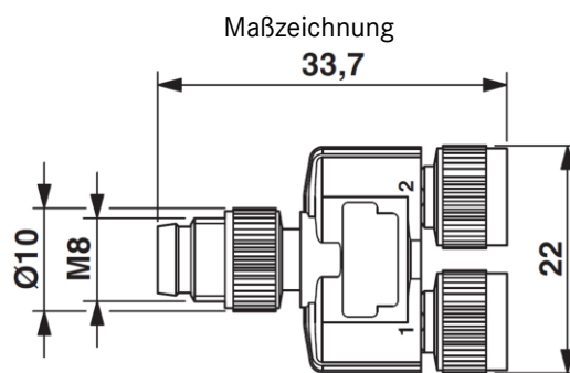
M8 Y-Verteiler
