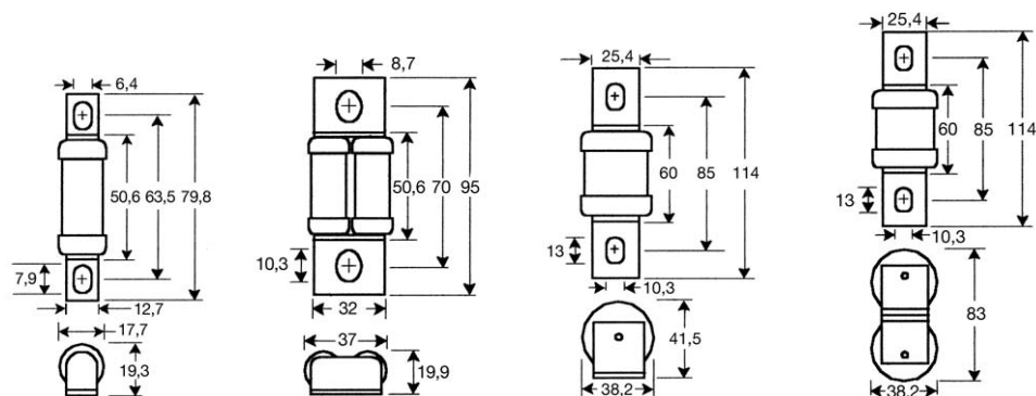
Fusibili tipo W-660GH Fuse type W-660GH
