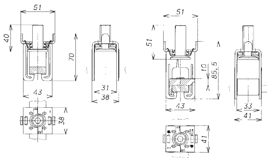
Morsetto 01319 - 01319 terminal
