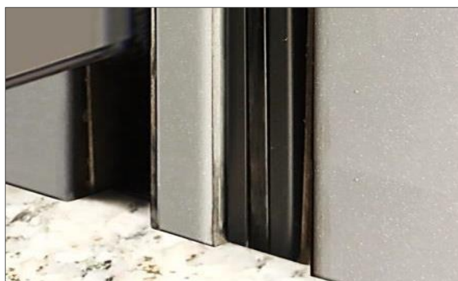
BPSLIM può essere incassata all'interno di una guida per tapparelle con larghezza minima 18 mm
