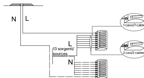
MAPA ROSONE CLOUD SP25 - schema cablaggio / wiring diagram
