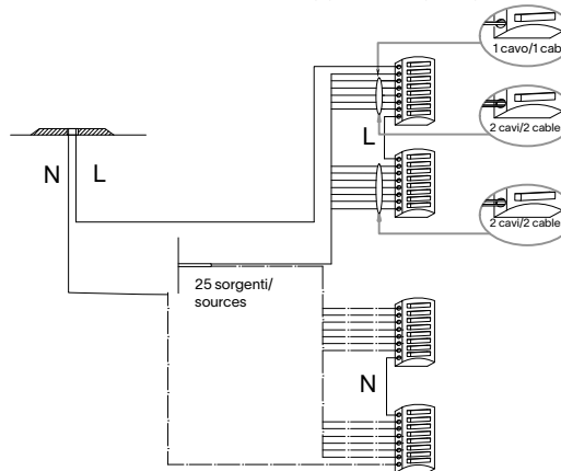
MAPA ROSONE CLOUD SP25 - schema cablaggio / wiring diagram
