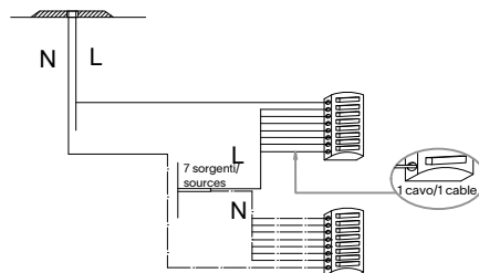
MAPA ROSONE CLOUD SP13 - schema cablaggio / wiring diagram
