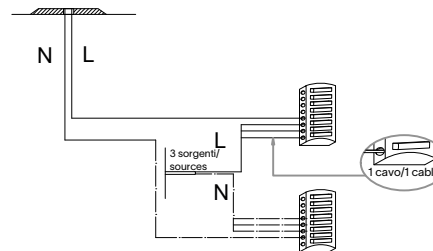
MAPA ROSONE CLOUD SP7 - schema cablaggio / wiring diagram
