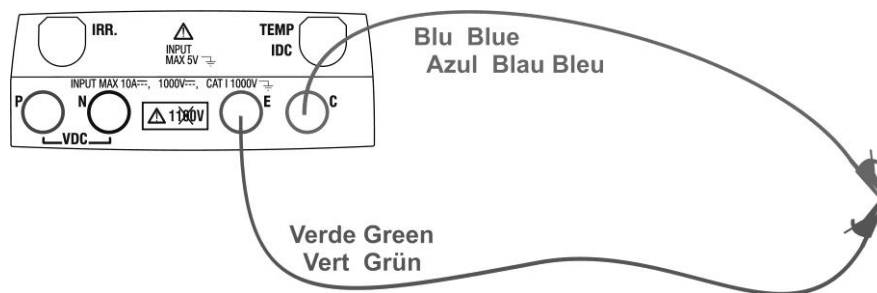
Fig. 13: Compensazione della resistenza dei cavi di misura
