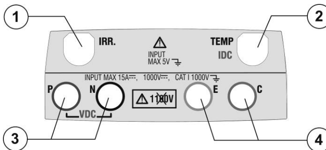
Fig. 2: Descrizione parte superiore dello strumento
