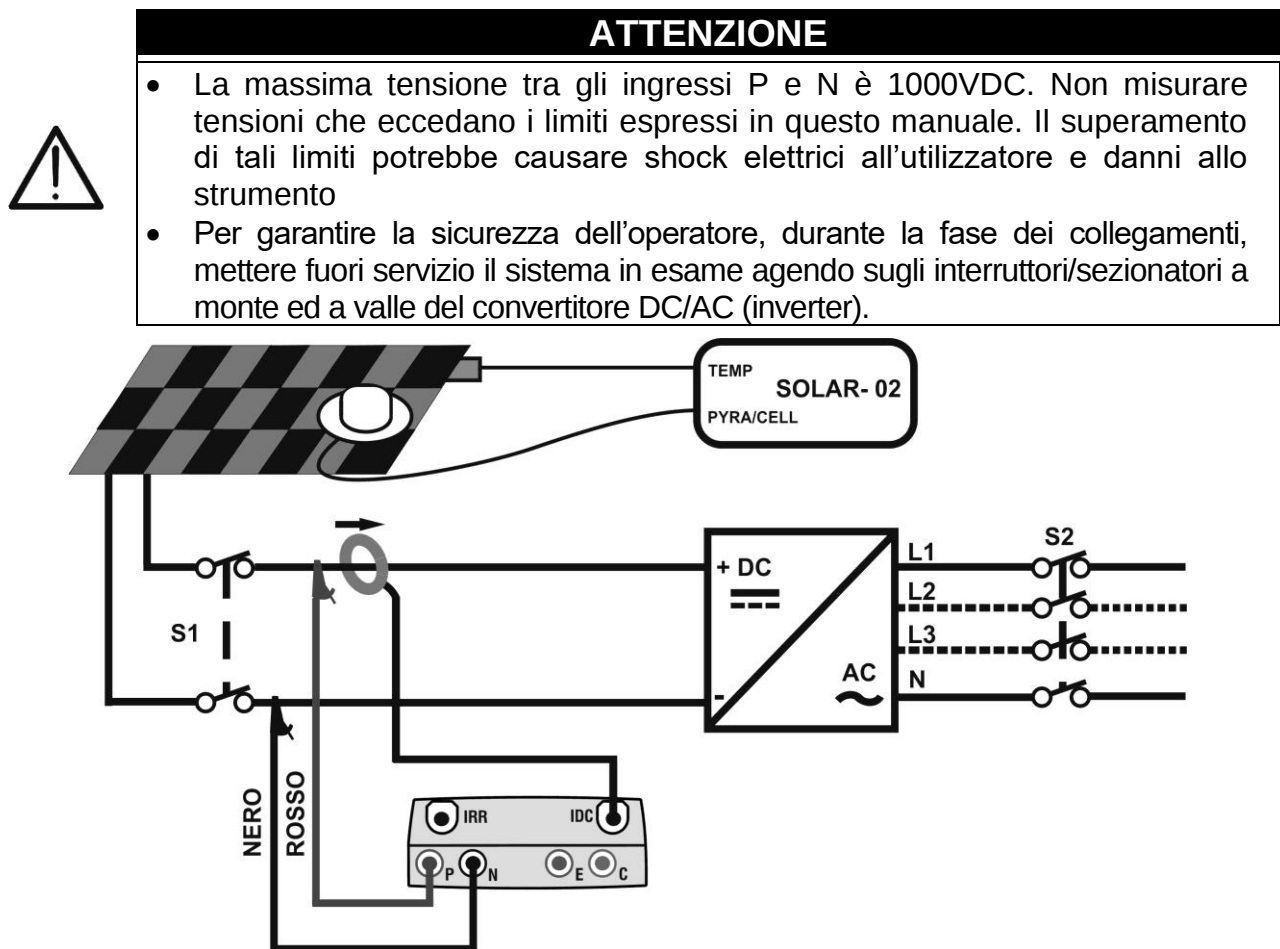
Fig. 4: Collegamento dello strumento per misura di efficienza su impianto FV
