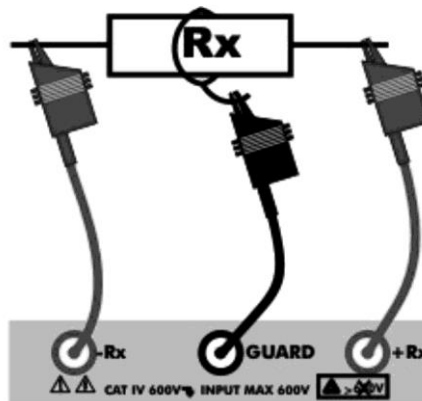
Fig. 4: Conexión del instrumento
