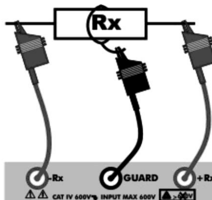
Fig. 6: Ligação do instrumento
