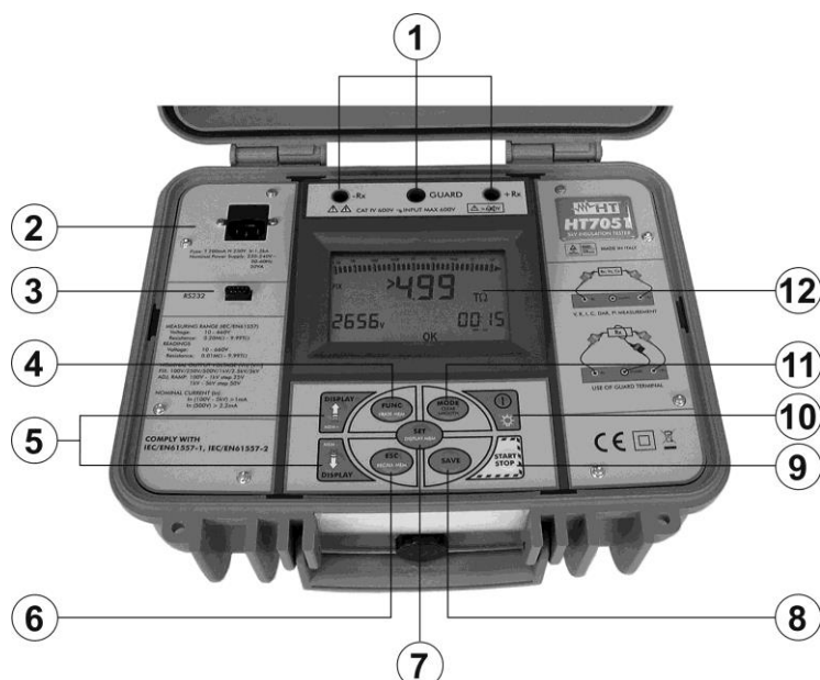
Fig. 1 : Description de l'instrument
