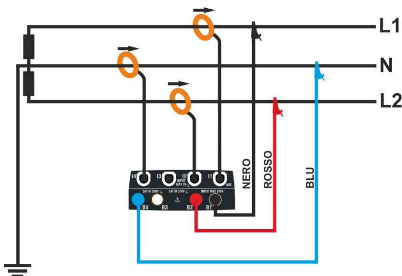
Fig. 17: Collegamento per misura su impianto Bifase 1φ-PresaCentrale – sistemi USA
