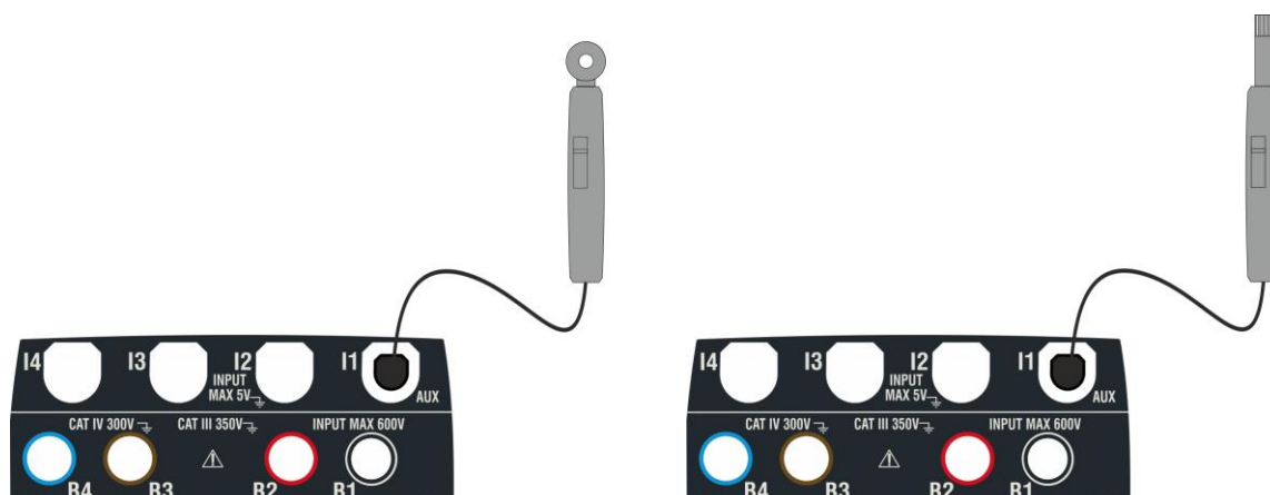
Fig. 8: Misura parametri ambientali con sonde esterne
