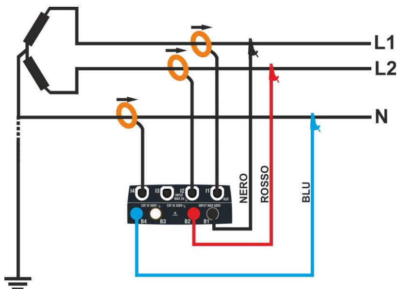
Fig. 15: Collegamento per misura su impianto Bifase 3φ-Y Aperta – sistemi USA
