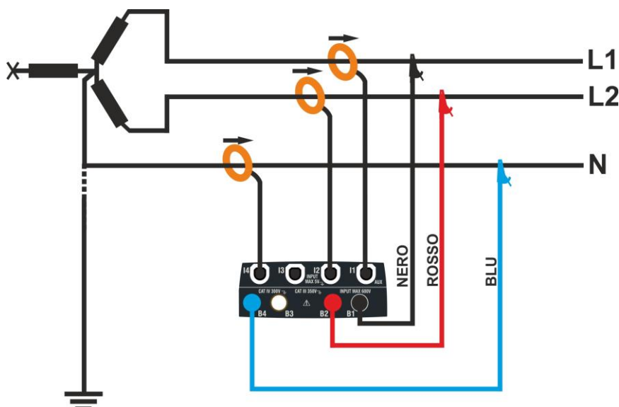
Fig. 16: Collegamento per misura su impianto Bifase 3φ-2EI. 1/2 – sistemi USA
