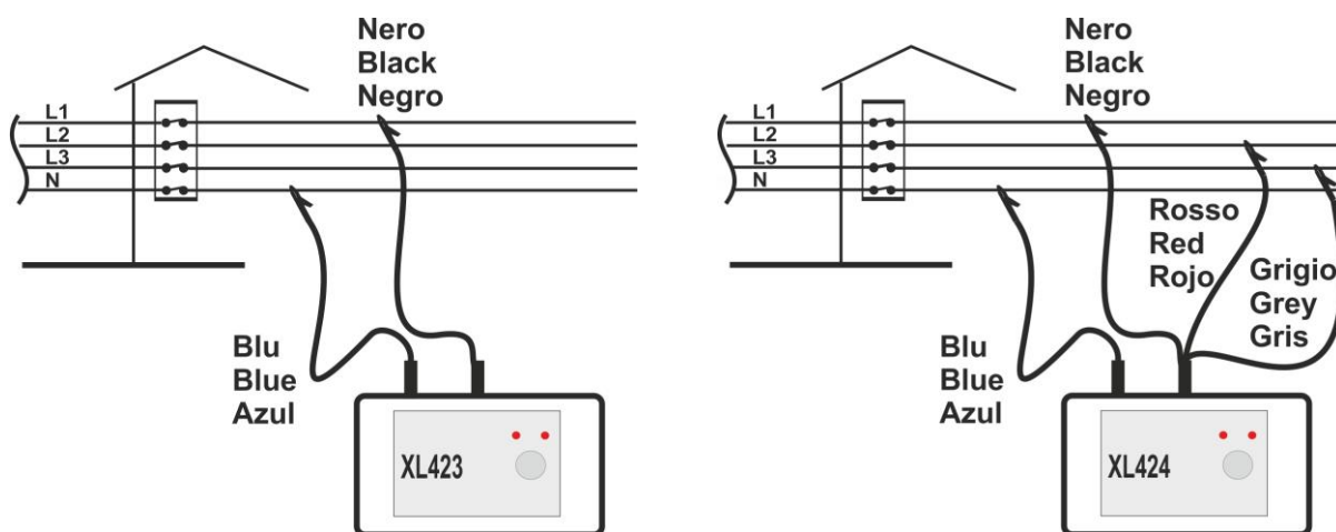
Fig. 3: Collegamento dello strumento in un sistema Trifase 4-fili
