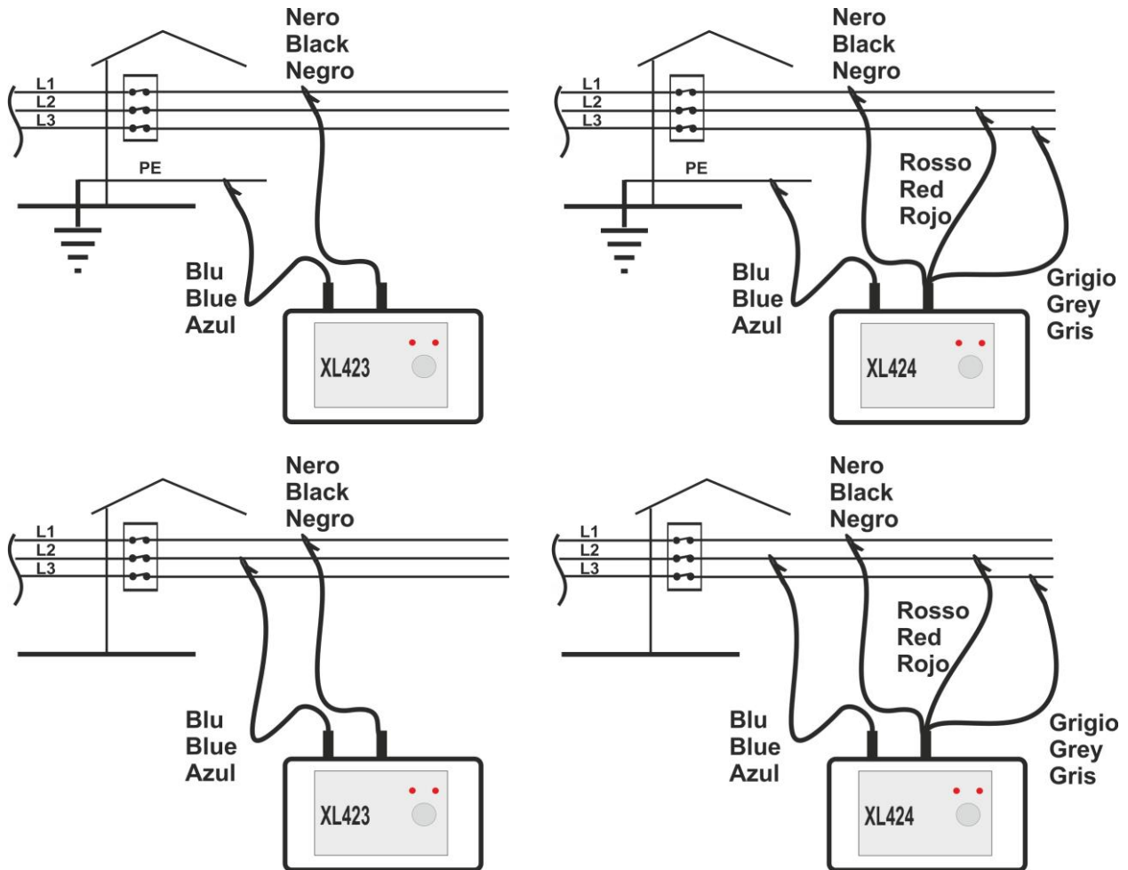
Fig. 4: Conexión del instrumento en un sistema Trifásico 3-cables
