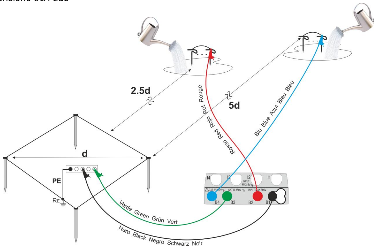
Fig. 53: Misura di terra per reti di terra di piccole dimensioni
