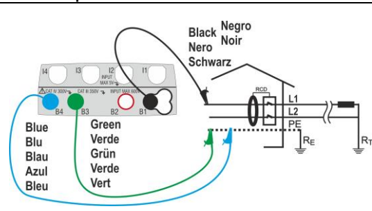
Fig. 11: Collegamento in sistema bifase senza neutro (no RCD tipo B/B+)
