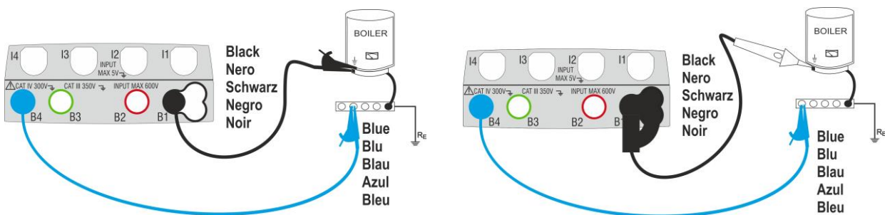
Fig. 6: Prova di continuità tramite cavi singoli e puntale remoto PR400
