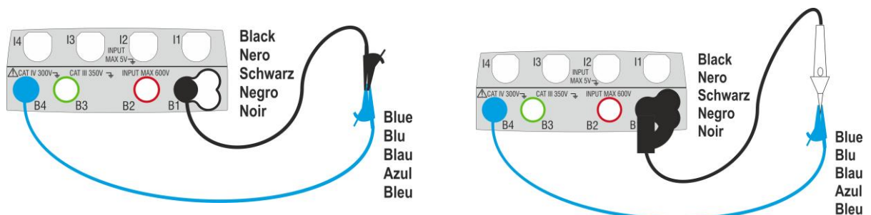
Fig. 7: Compensazione della resistenza dei cavi singoli e del puntale remoto
