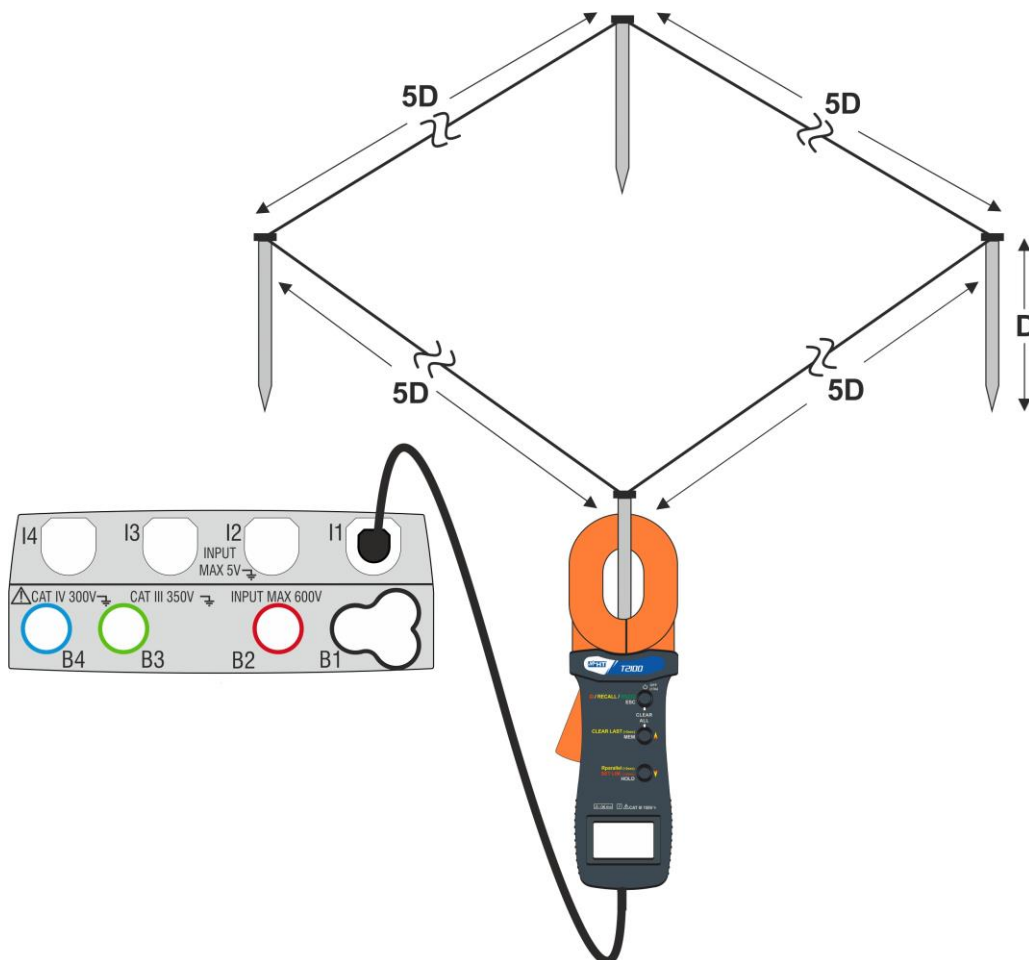
Fig. 31: Misura resistenza dispersori singoli con pinza T2100
