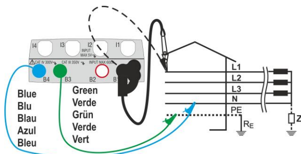
Fig. 22: Misura L-PE in sistemi IT con cavi singoli e puntale remoto
