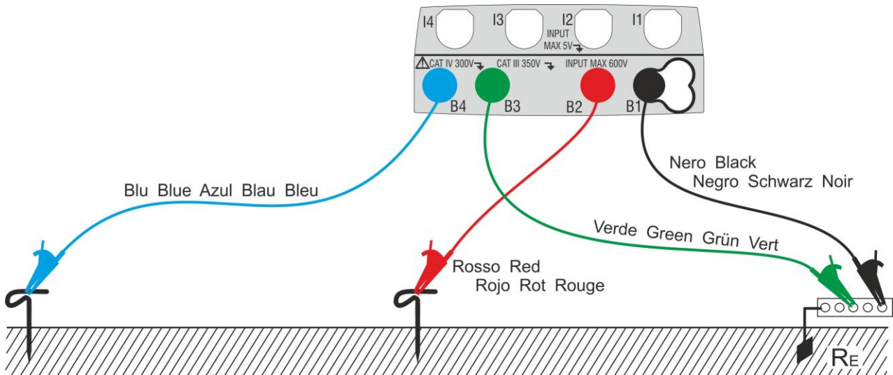
Fig. 27: Misura della resistenza di terra a 3 fili
