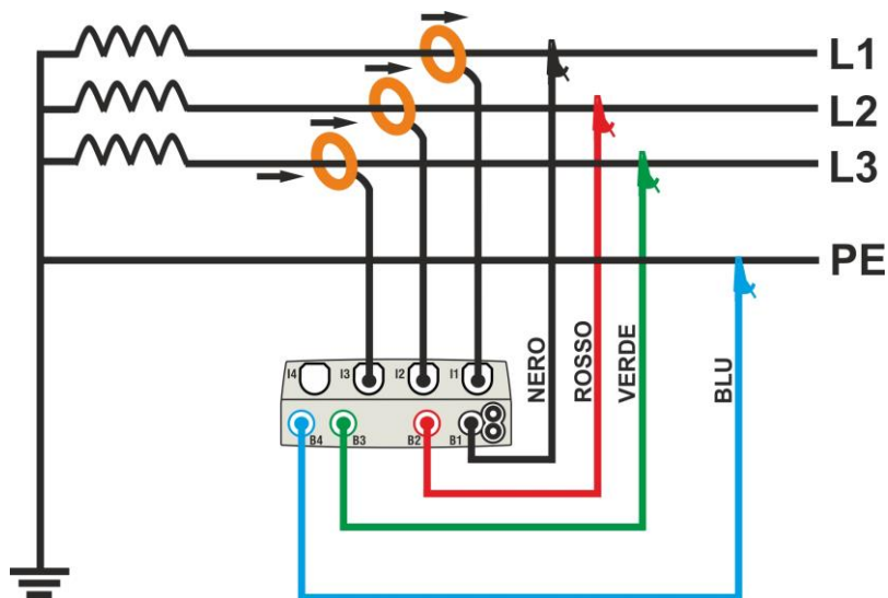
Fig. 38: Collegamento per misura su impianto Trifase 3φ-3FILI
