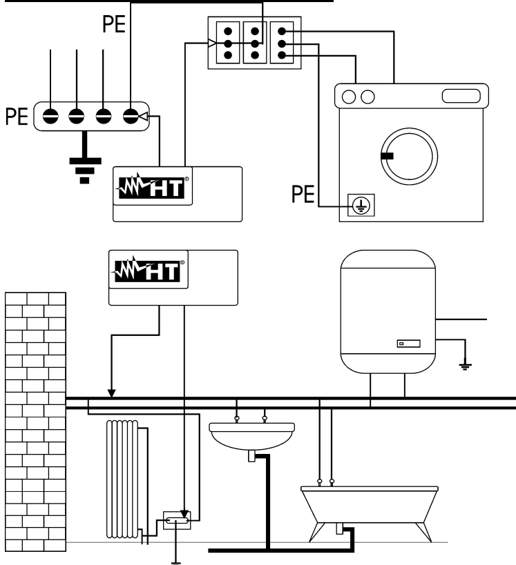
Fig. 50: Esempi di misure di continuità dei conduttori
