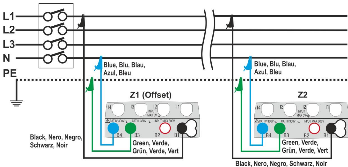
Fig. 34: Collegamento strumento per misura caduta di tensione in modo L-N
