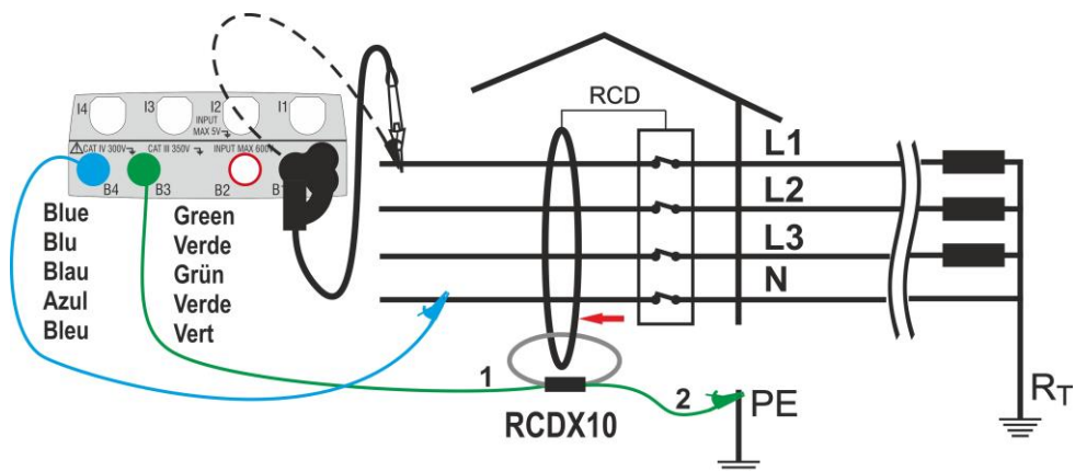
Fig. 16: Collegamento a RCD con toroide separato con accessorio opzionale RCDX10
