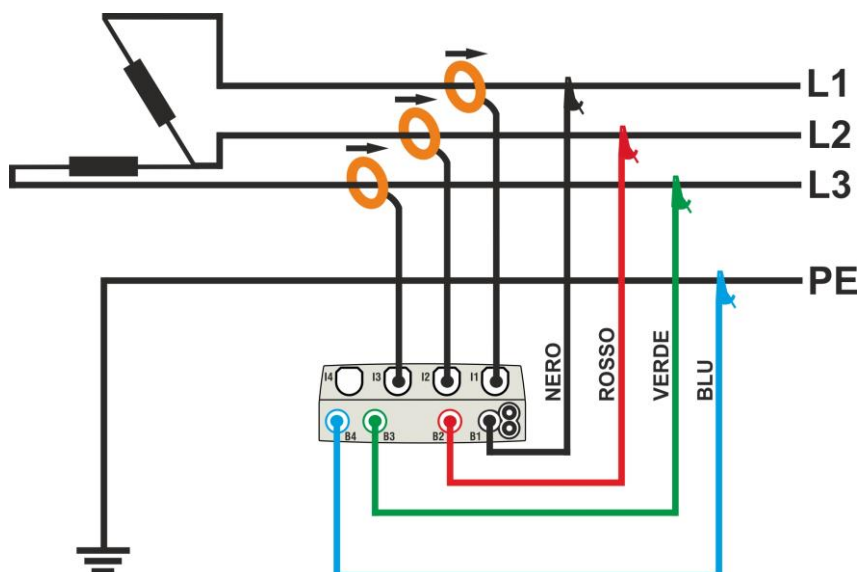
Fig. 41: Collegamento per misura su impianto Trifase 3 \phi - \Delta Aperto – sistemi USA
