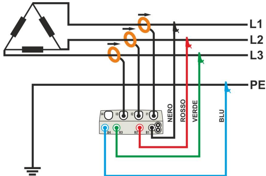
Fig. 39: Collegamento per misura su impianto Trifase 3 \phi -ARON
