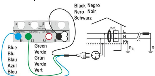
Fig. 10: Collegamento in sistema monofase tramite spina shuko
