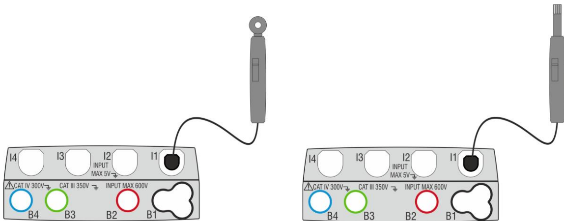
Fig. 32: Misura parametri ambientali con sonde esterne
