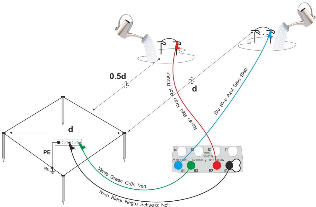
Fig. 54: Misura di terra per reti di terra di grandi dimensioni
