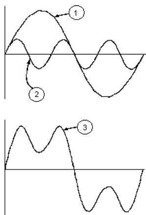
Fig. 57: Effetto della sovrapposizione di due frequenze multiple l'una dell'altra
