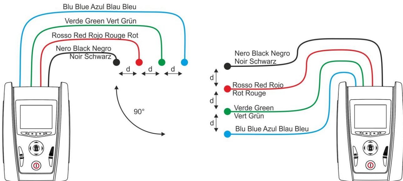
Fig. 55: Misura della resistività del terreno
