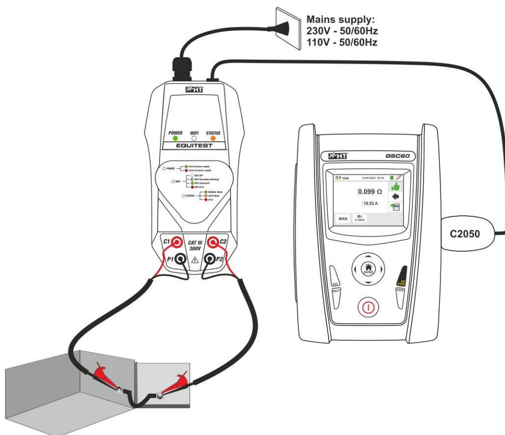
Fig. 33: Misura continuità conduttori di protezione con accessorio EQUITEST
