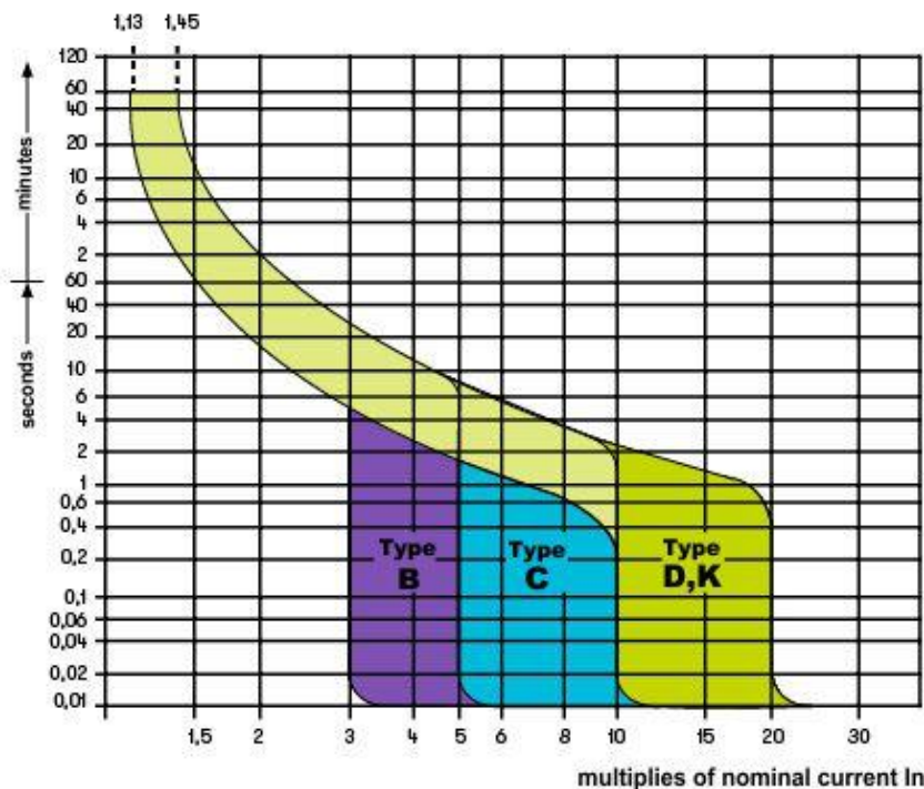
Fig. 52: Esempio di curve di intervento protezioni magnetotermiche (MCB)
