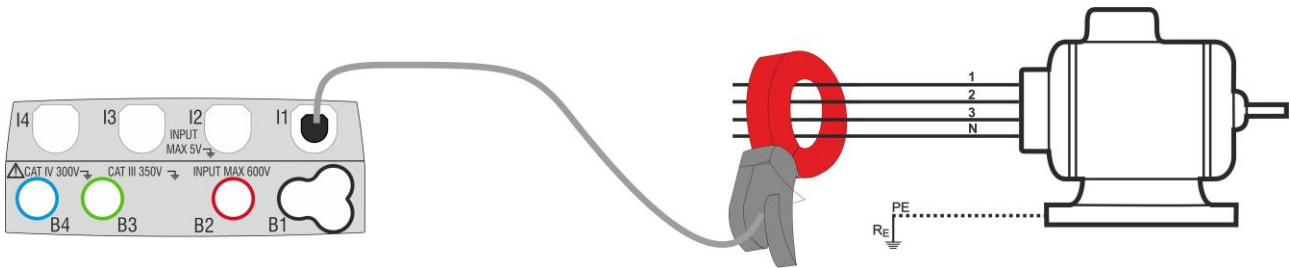
Fig. 25: Misurazione indiretta della corrente di dispersione in impianti trifase
