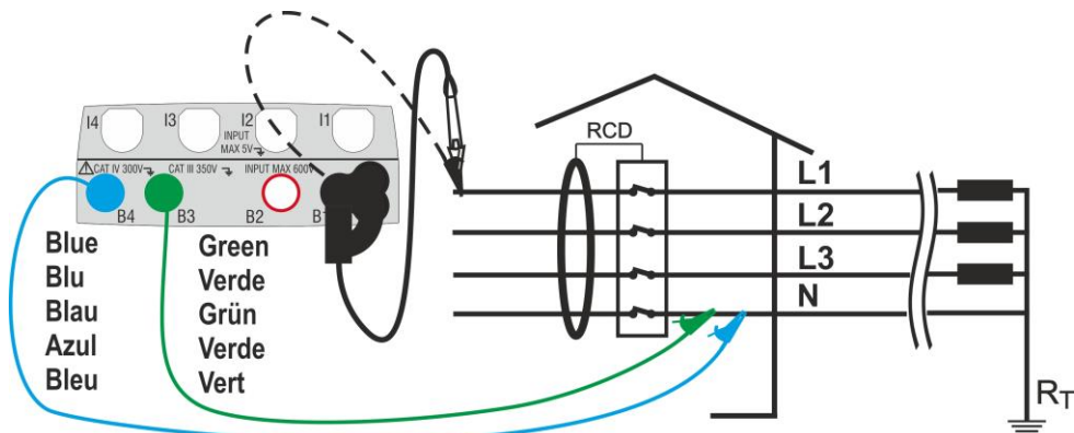
Fig. 14: Collegamento in sistema trifase (no PE) con cavi e puntale remoto (no RCD tipo B/B+)
