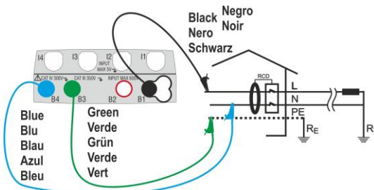
Fig. 12: Collegamento in sistema monofase con cavi singoli e puntale remoto
