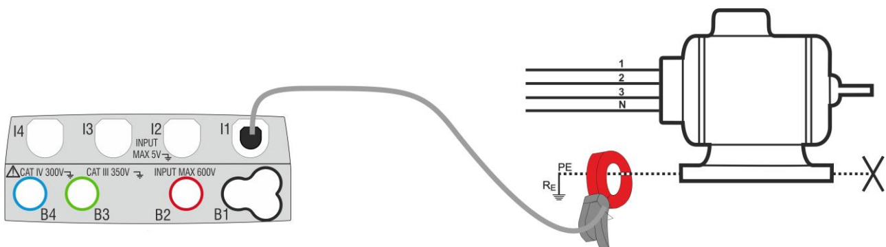
Fig. 26: Misurazione diretta della corrente di dispersione in impianti trifase
