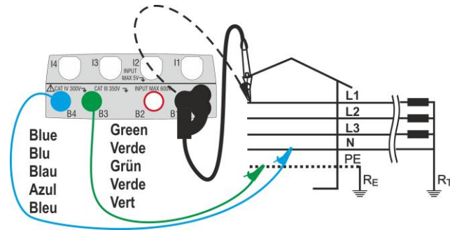
Fig. 19: Misura L-N/L-PE in impianti trifase con cavi singoli e puntale remoto
