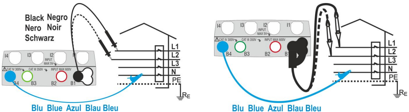
Fig. 24: Verifica del senso ciclico delle fasi 2T con terminale e puntale remoto
