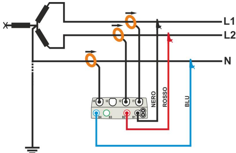
Fig. 43: Collegamento per misura su impianto Bifase 3φ-2EI. 1/2 – sistemi USA
