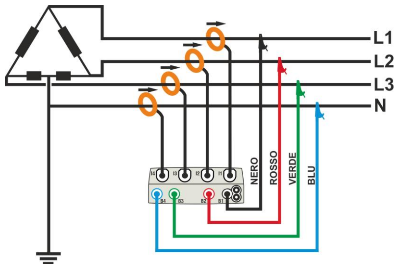
Fig. 40: Collegamento per misura su impianto Trifase 3 \phi -High Leg – sistemi USA
