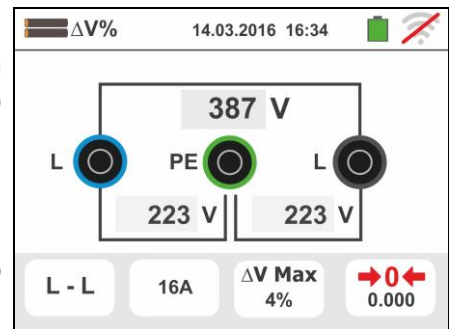
Fig. 35: Collegamento strumento per misura caduta di tensione in modo L-L
