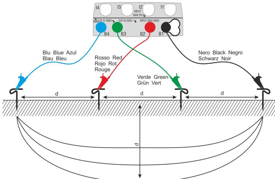
Fig. 30: Misura della resistività del terreno
