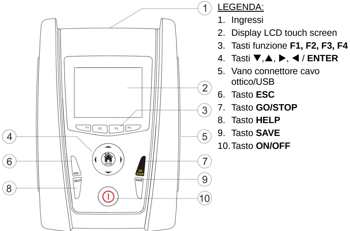
Fig. 1: Descrizione parte frontale dello strumento
