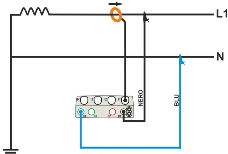
Fig. 36: Collegamento per misura su impianto Monofase 1φ-2FILI
