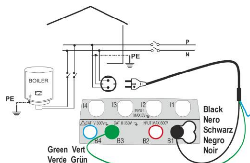
Fig. 9: Verifica dell'isolamento tramite spina shuko
