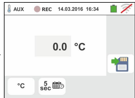
Fig. 32: Misura parametri ambientali con sonde esterne
