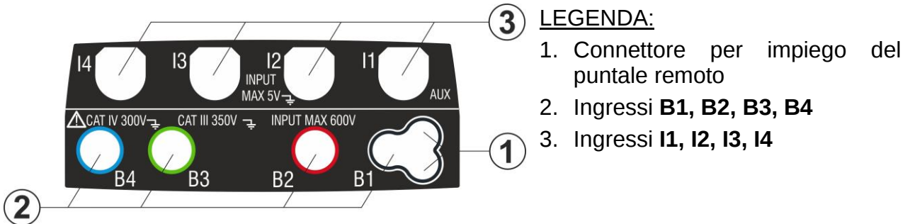
Fig. 2: Descrizione parte superiore dello strumento
