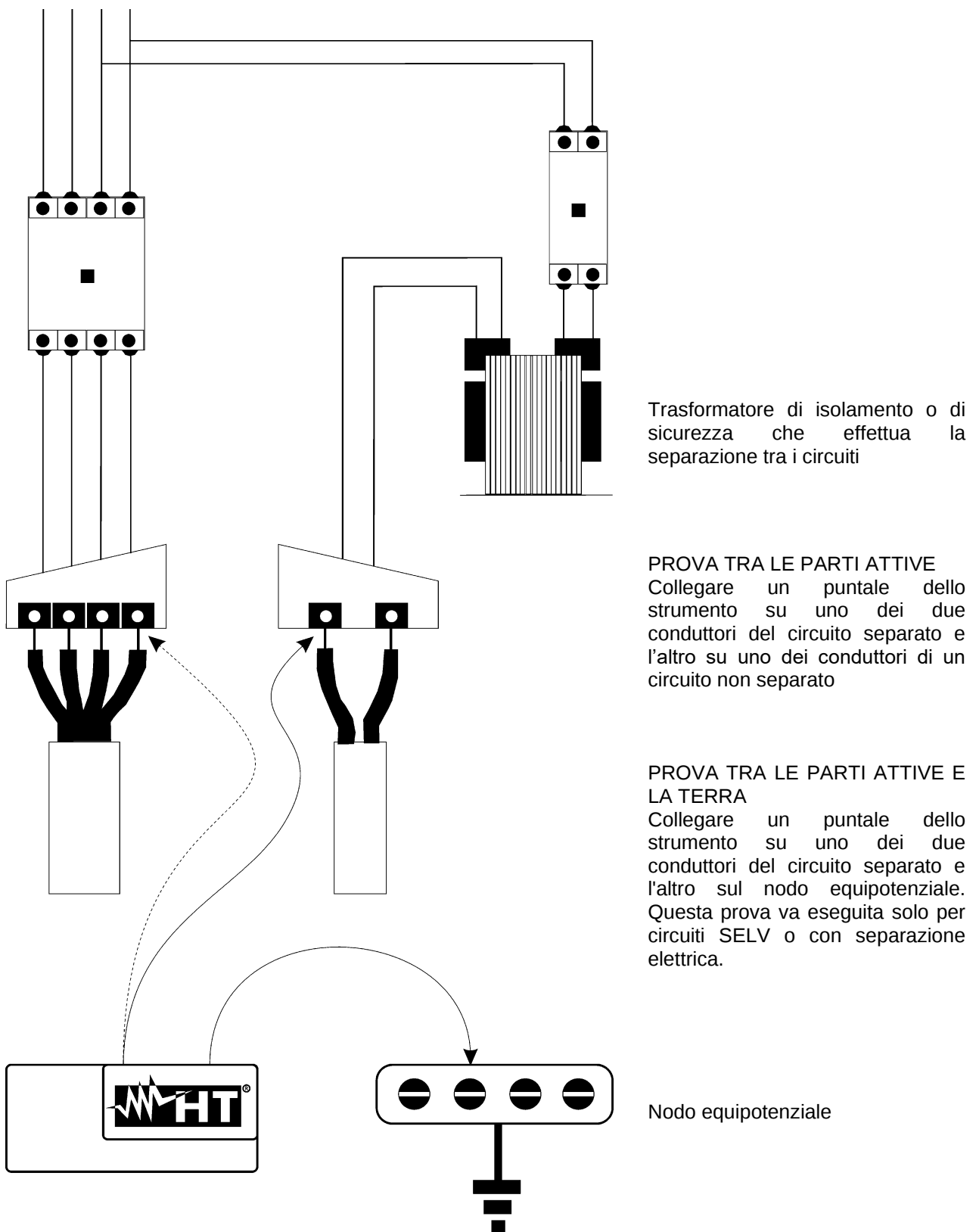
Fig. 51: Misure di separazione tra circuiti in un impianto
