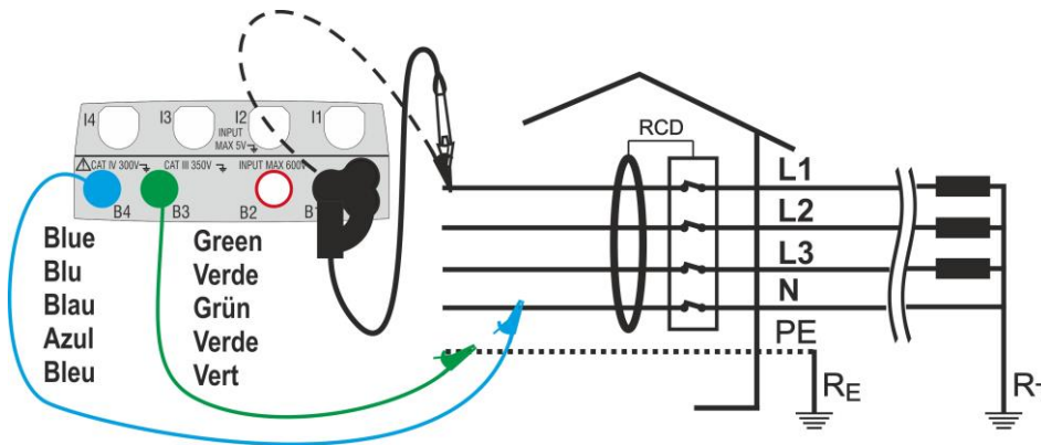
Fig. 13: Collegamento in sistema trifase con cavi singoli e puntale remoto
