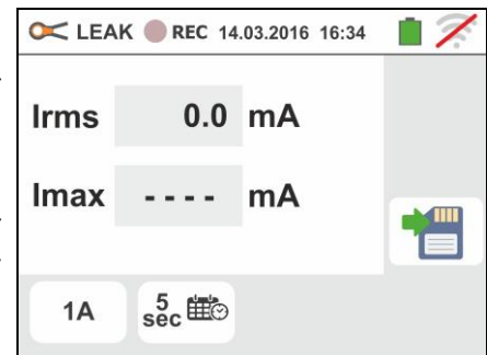
Fig. 26: Misurazione diretta della corrente di dispersione in impianti trifase
