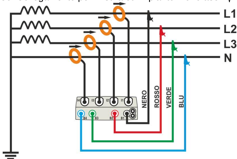
Fig. 37: Collegamento per misura su impianto Trifase 3φ-4FILI
