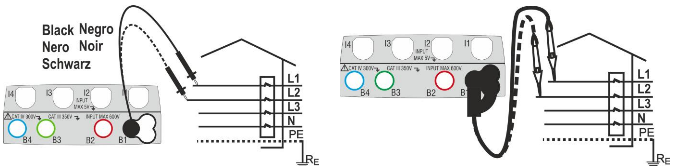
Fig. 23: Verifica del senso ciclico delle fasi 1T con terminale e puntale remoto
