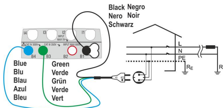
Fig. 17: Misura L-N/L-PE in impianti monofase/bifase 230V tramite spina shuko
