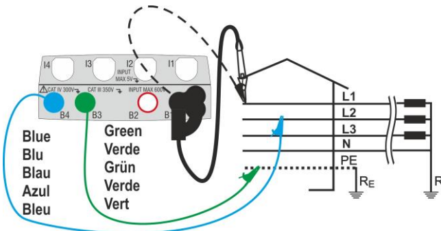
Fig. 20: Misura L-L in impianti trifase con cavi singoli e puntale remoto
