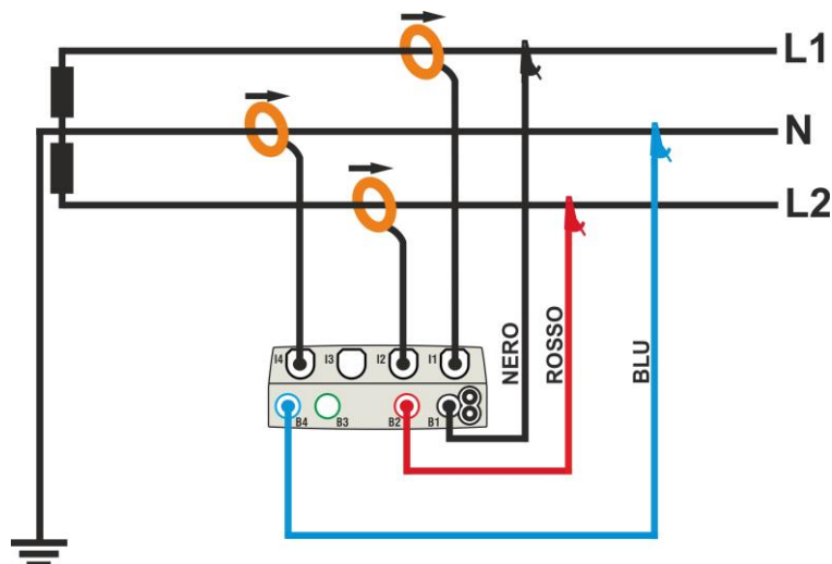
Fig. 44: Collegamento per misura su impianto Bifase 1φ-PresaCentrale – sistemi USA
