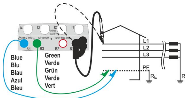
Fig. 21: Misura L-PE/L-N in impianti trifase 3 fili (no N) con cavi singoli e puntale remoto
