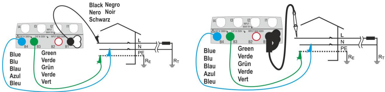
Fig. 18: Misura L-N/L-PE in impianti monofase/bifase con cavi e puntale remoto
