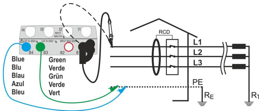
Fig. 15: Collegamento sistema trifase (no N) con cavi e puntale remoto (no RCD tipo B/B+)
