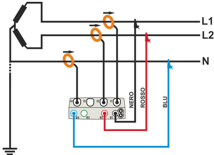
Fig. 42: Collegamento per misura su impianto Bifase 3φ-Y Aperta – sistemi USA
