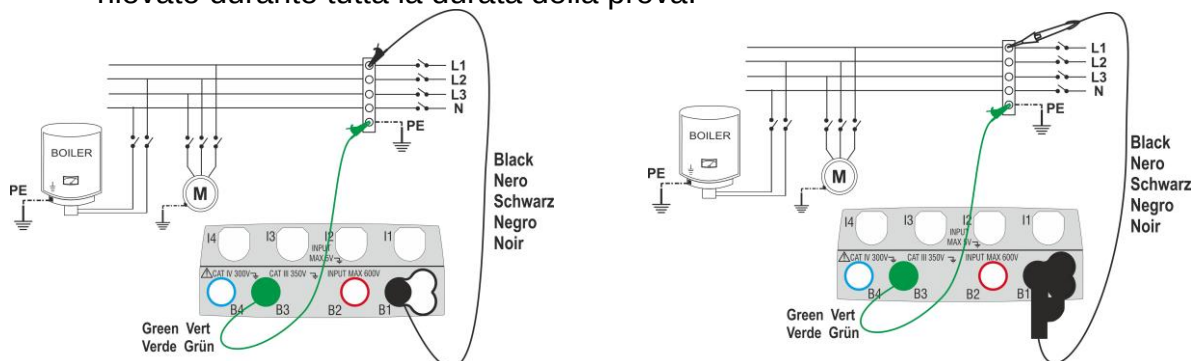
Fig. 8: Verifica dell'isolamento tramite cavi singoli e puntale remoto
