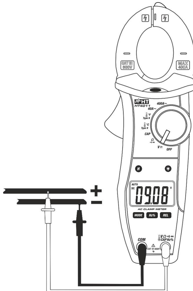
Fig. 3: Uso da pinça na medição de Tensões CC
