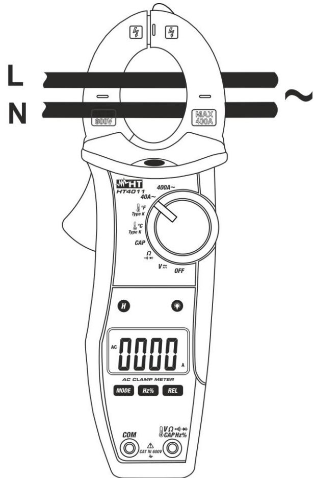
Fig. 10 : Utilisation de la pince pour mesure de courant CA
