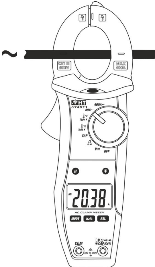
Abb. 10: Verwendung der Zange für Wechselstrommessung
