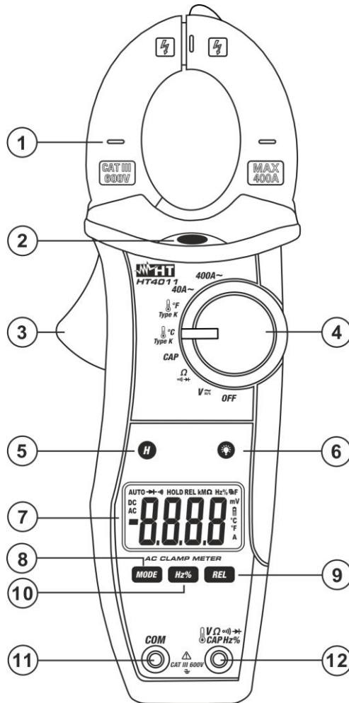
Fig. 1 : Description de l'instrument
