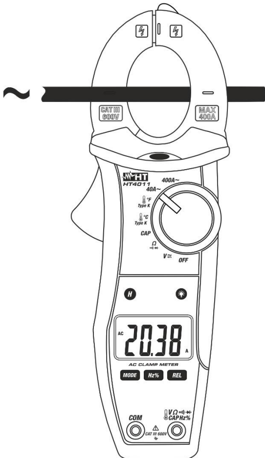
Fig. 10: Uso da pinça para medições de corrente CA
