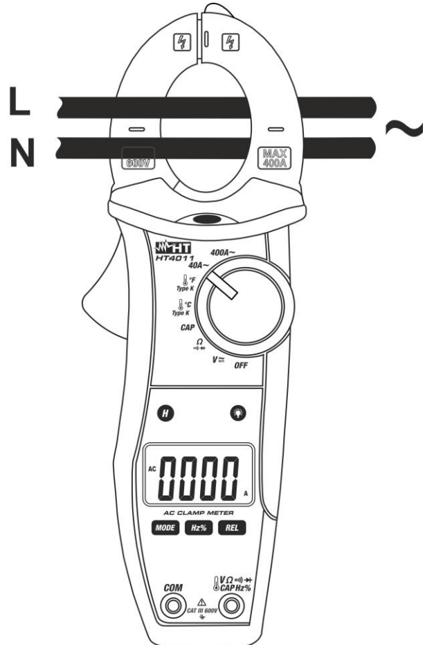
Abb. 10: Verwendung der Zange für Wechselstrommessung
