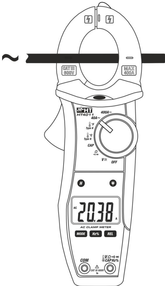
Fig. 10 : Utilisation de la pince pour mesure de courant CA
