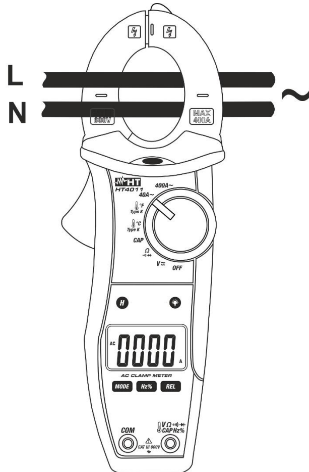
Fig. 10: Uso da pinça para medições de corrente CA
