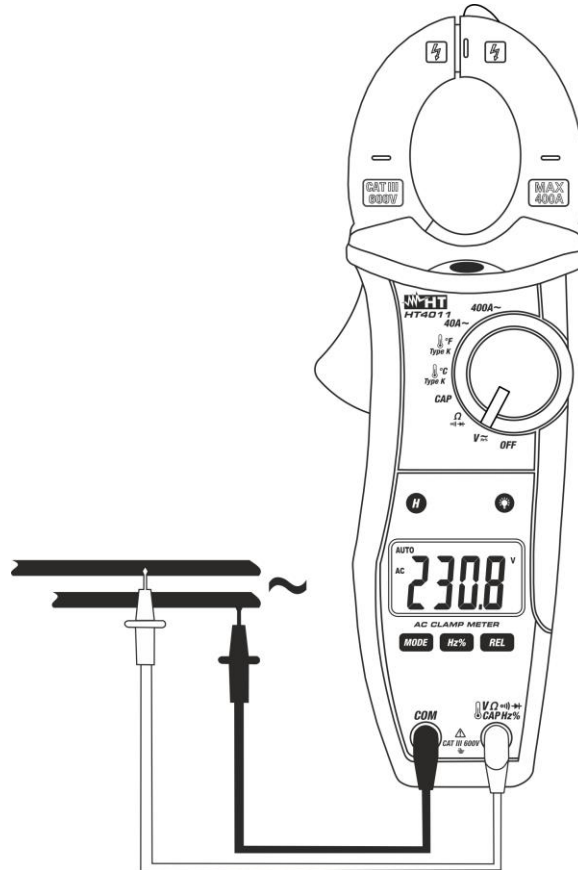
Abb. 4: Verwendung der Zange für Wechselspannungsmessung
