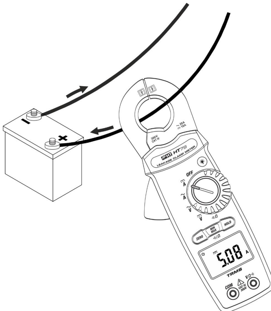
Fig. 8: Uso do instrumento para medir Correntes CC
