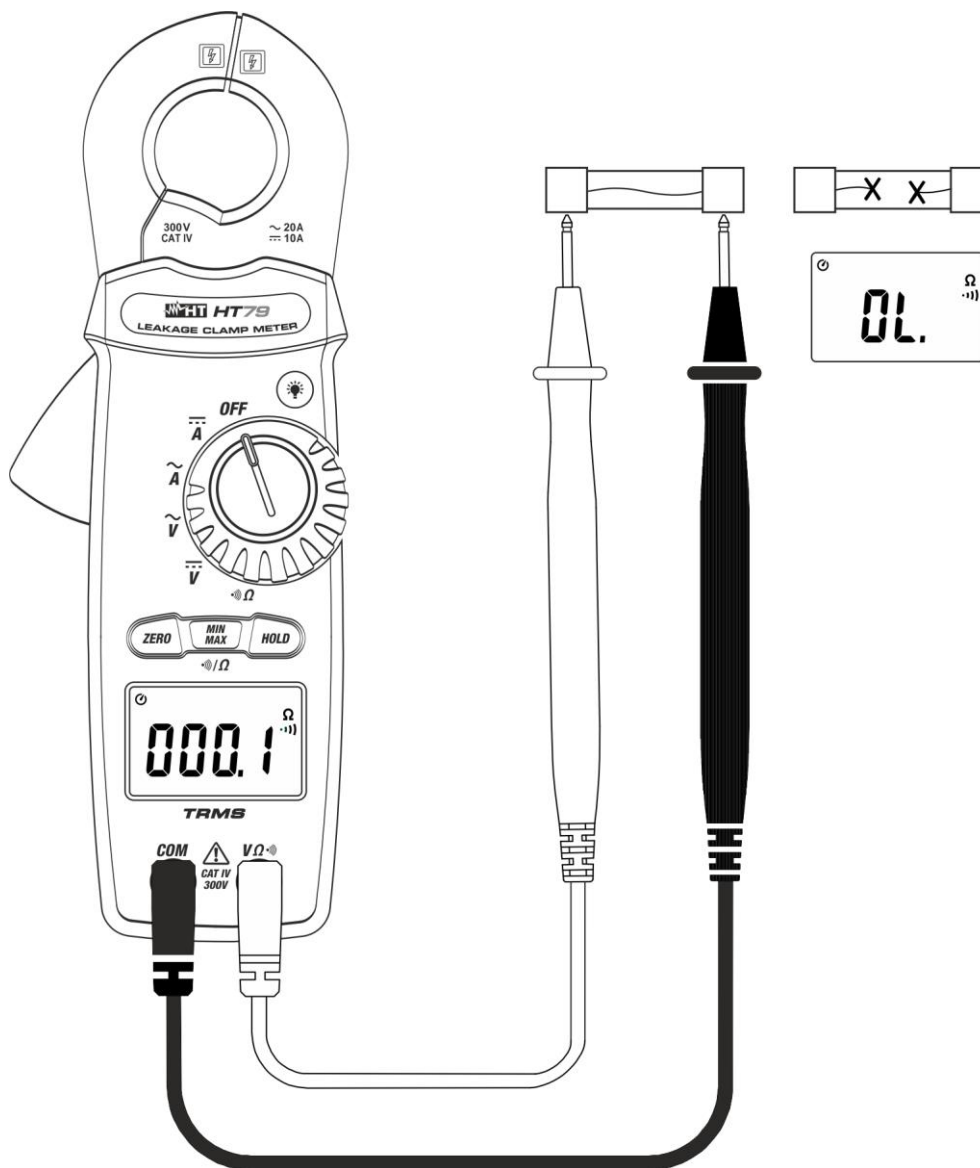
Fig. 7: Uso del instrumento para la prueba de continuidad
