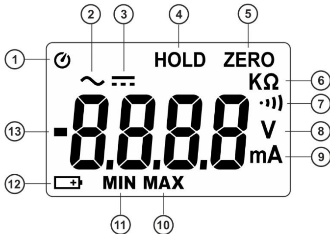
Fig. 3: Descrição d display
