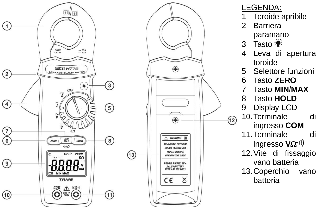
Fig. 1: Descrizione dello strumento
