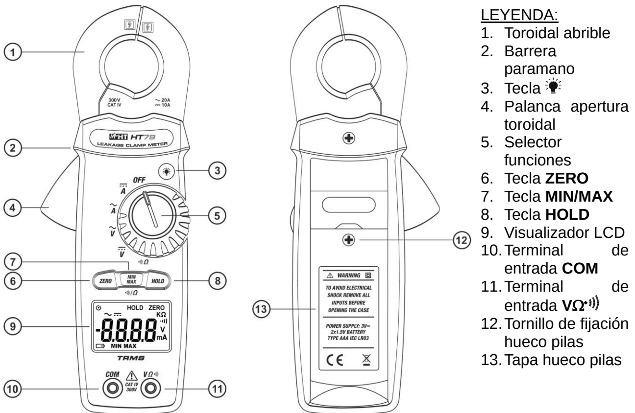
Fig. 1: Descripción del instrumento
