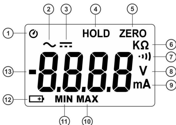
Fig. 3: Descripción del visualizador
