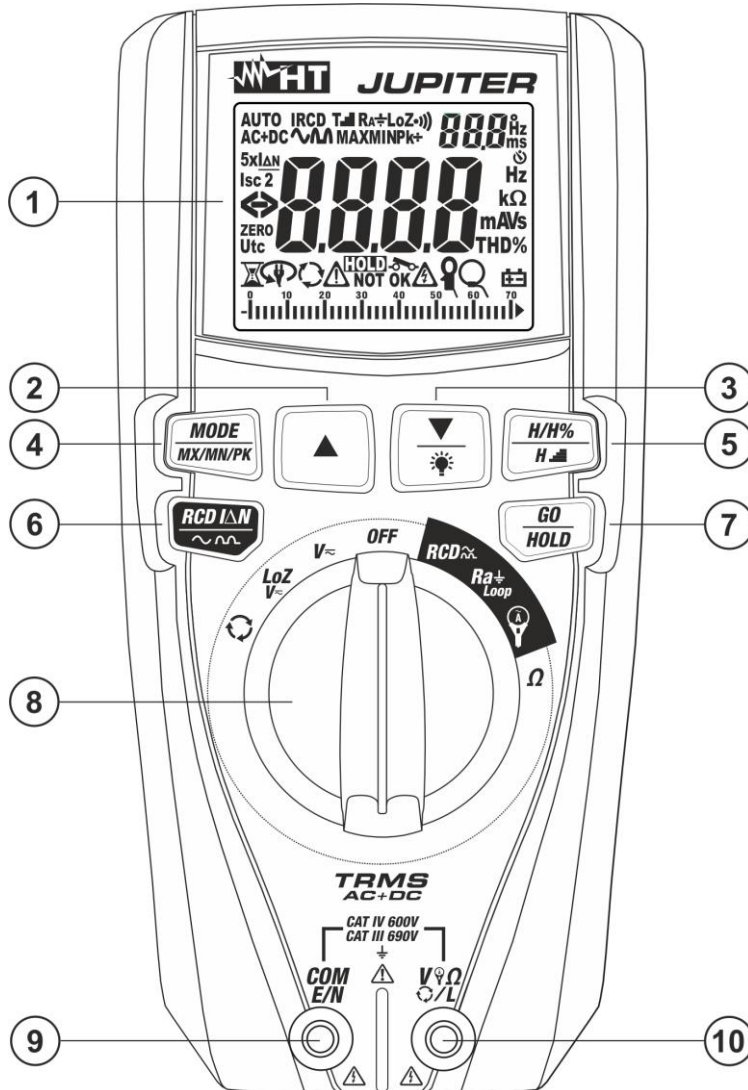
Fig. 1: Descrizione dello strumento
