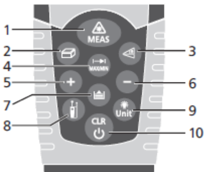
Fig. 1: Descrição do instrumento
