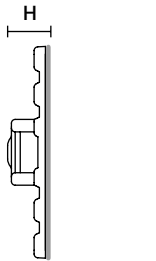
Basetta flessibile adesiva FMB4APT-A (vista laterale)
