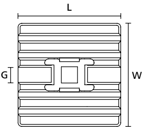
Basetta flessibile adesiva FMB4APT-A (vista planimetrica)
