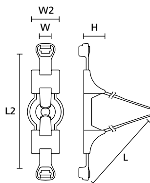
DHDM con fascetta (L = lunghezza della parte piatta)
