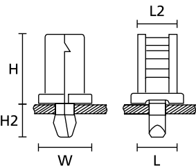
Supporto con rivetto TY5K1
