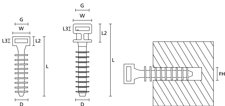
Supporti a tassello serie LOK01 (vista frontale).
