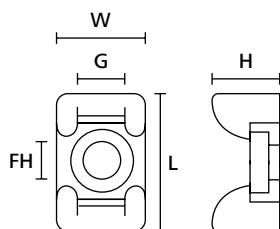
Basette KR6G5, KR8G5 e CTM (vista dall'alto)
