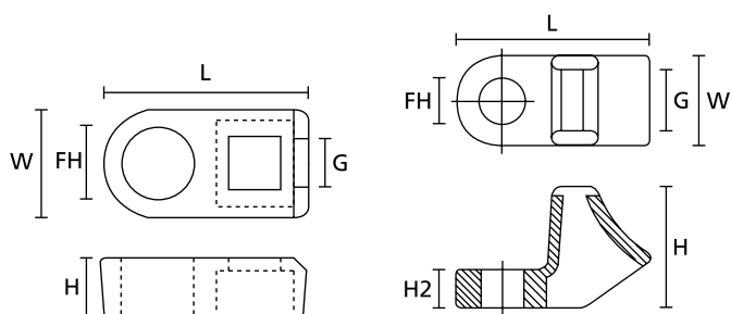
Supporto FH (vista dall'alto e laterale)
