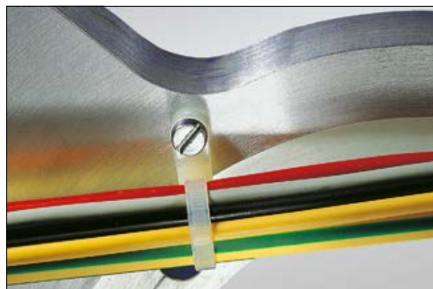
Le fascette con testa di fissaggio ad occhiello possono essere facilmente fissate ad un pannello.
