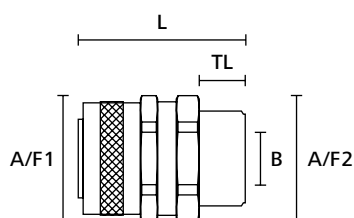
Raccordo girevole diritto con filetto maschio
