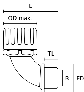
Raccordo HelGuard curvato a 90° con filetto maschio
