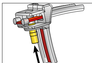
Testa della fascetta KR prima della chiusura
