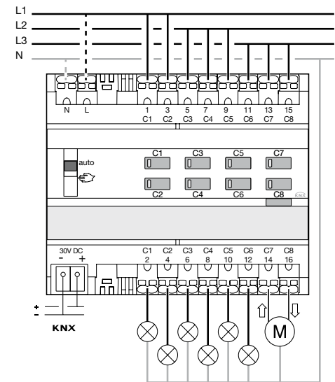
Afb. 2: apparaat aansluiten
