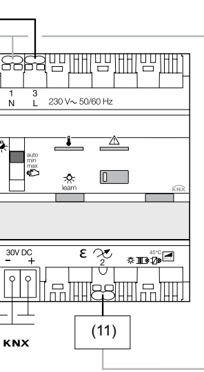
Afb. 3: apparaat aansluiten
