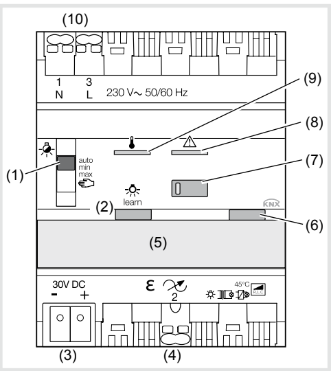
Afb. 1: overzicht apparaten
