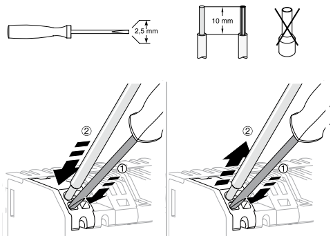
Afb. 2: installatie/deinstallatie met steekklemmen
