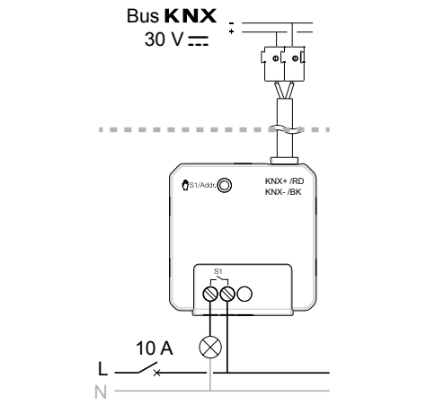
Afb. 3: apparaat aansluiten 1-voudig
