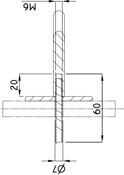
SEZIONE A-A SCALA 1 / 2
