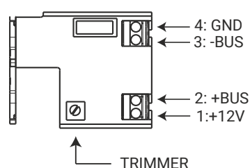
Morsetti inseritore
