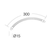
Giunto angolare Flex - Slim 3
