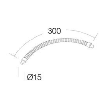
Giunto angolare Flex - Slim 3
