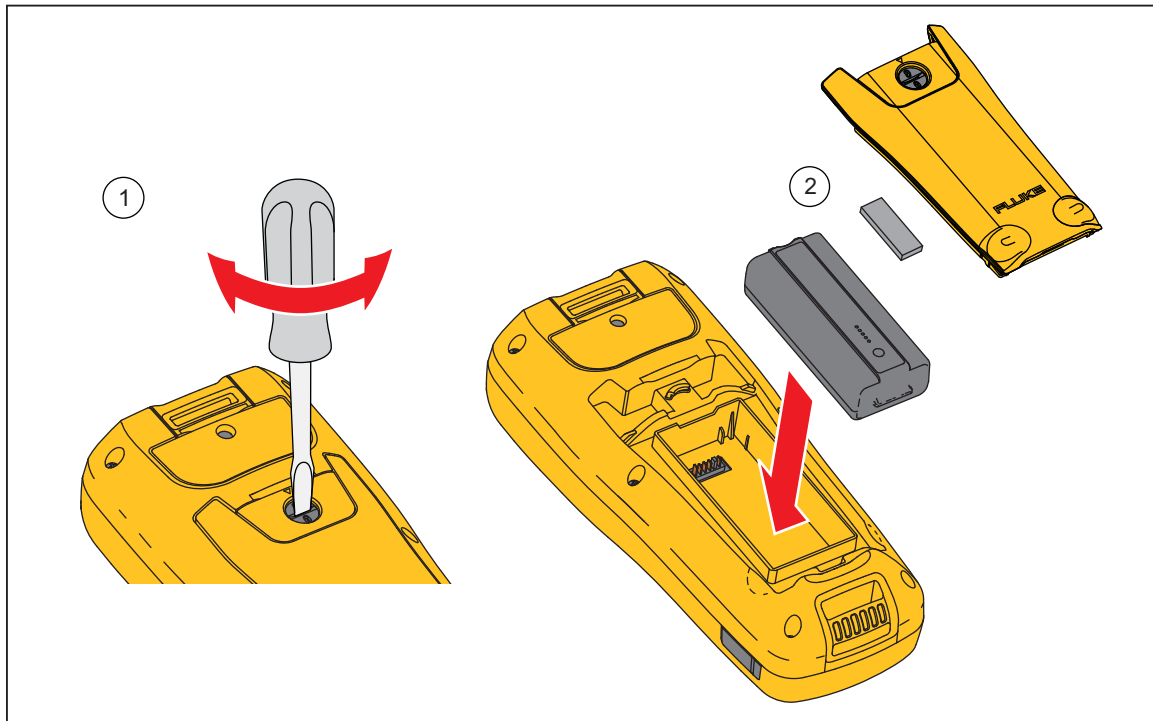
Figura 6-1. Installazione o sostituzione del pacco batterie
