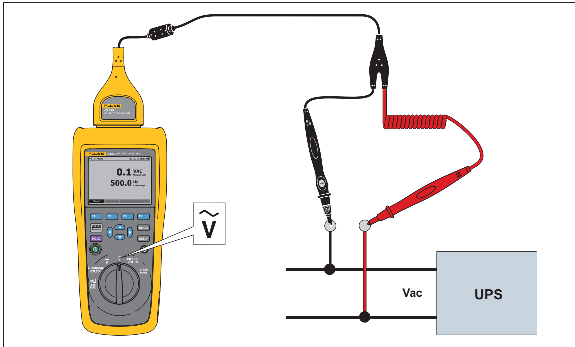
Figura 3-4. Misurazione della tensione c.a.
