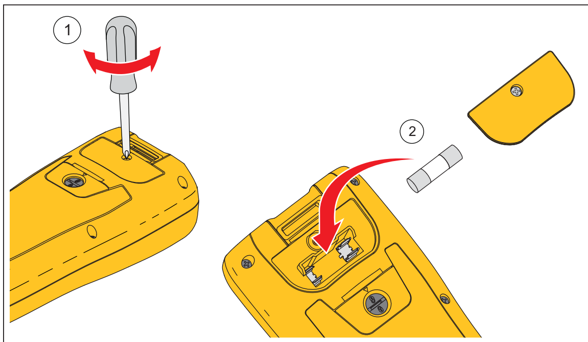
Figura 6-2. Sostituzione del fusibile
