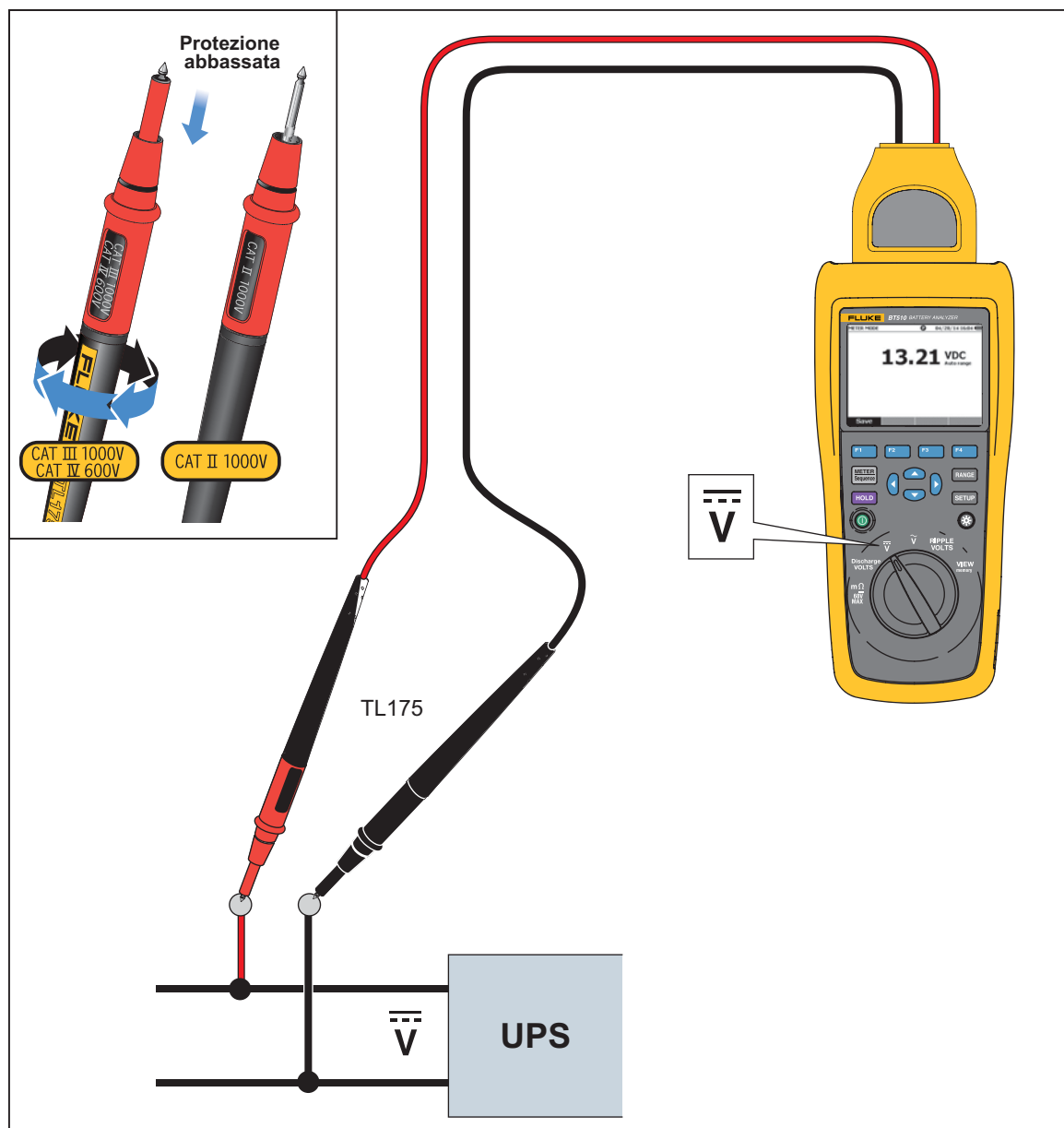
Figura 3-5. Misurazione della tensione c.c. con TL175
