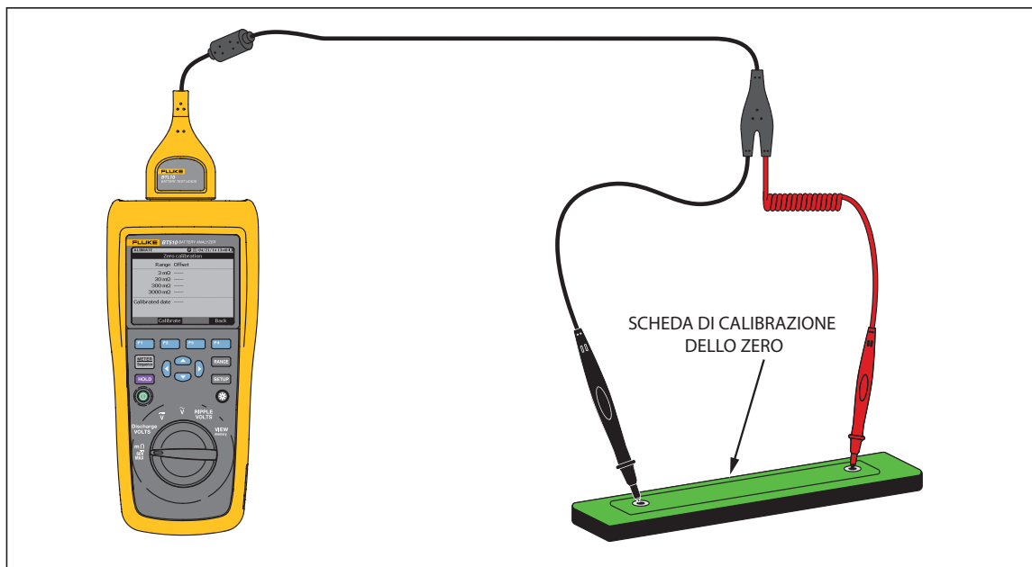
Figure 6-4. Configurazione della calibrazione dello zero
