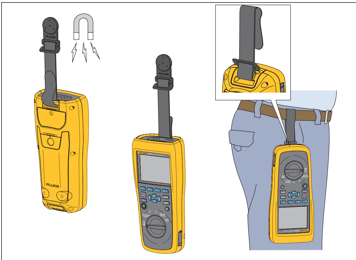
Figura 2-2. Cinghia
