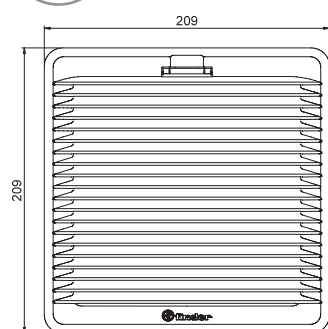
Tipo 7F.xx.x.xxx.4250 Morsetti Push-in
