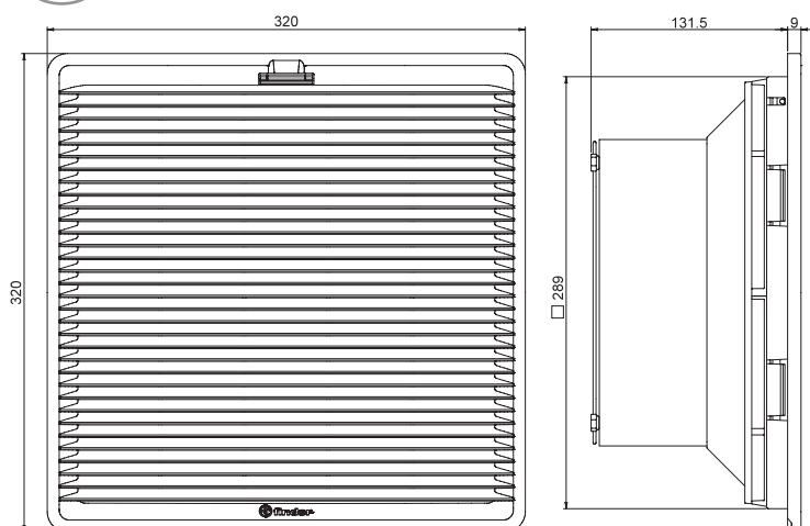
Tipo 7F.xx.x.xxx.5700 Morsetti Push-in
