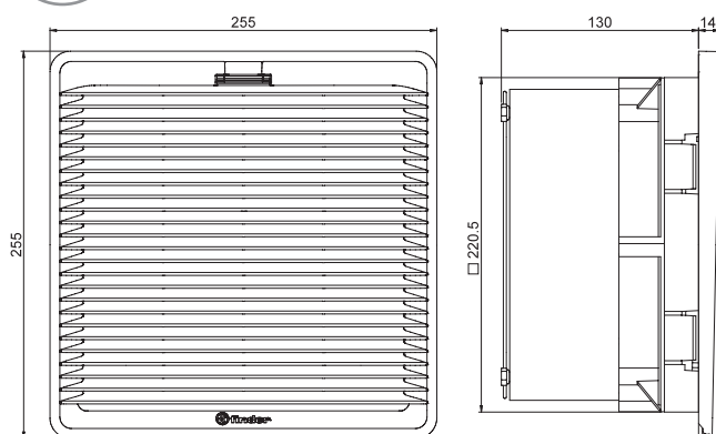
Tipo 7F.xx.x.xxx.5550 Morsetti Push-in
