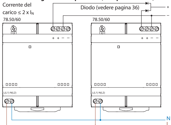
Collegamento in parallelo (solo per 78.50/60)
