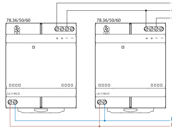
Collegamento in serie
