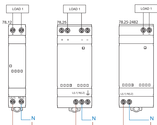
Collegamento a doppia polarità
