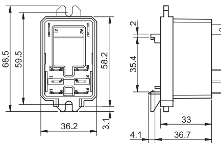
066.07 con relè
