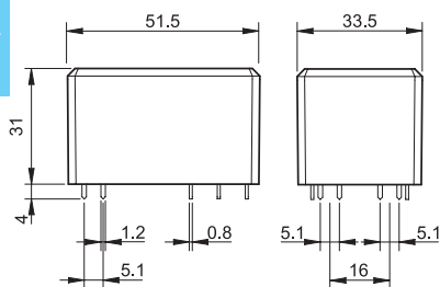
Tipo 66.22-x300
