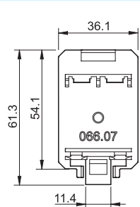
Adattatore barra 35 mm (EN 60715) in testa per 66.82.x.xxx.xx00
