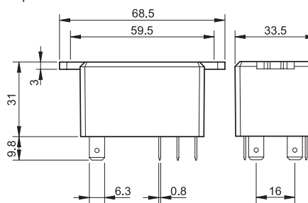
Tipo 66.82
