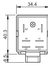
Adattatore barra 35 mm (EN 60715) in testa per relè tipo 65.31.x.xxx.xxx9
