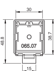
Adattatore barra 35 mm (EN 60715) in testa per relè tipo 65.31.x.xxx.xxx9
