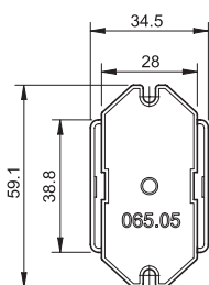
Adattatore con aletta in testa per relè tipo 65.31.x.xxx.xxx9
