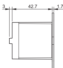
Adattatore con aletta in testa per relè tipo 65.31.x.xxx.xxx9
