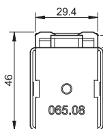
Adattatore barra 35 mm (EN 60715) sul retro per relè tipo 65.31.x.xxx.xxx9
