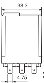
Tipo 62.33 62.33-4300
