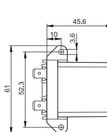
062.10 con relè
