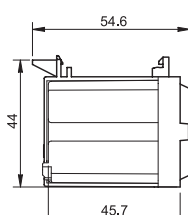
062.08 con relè
