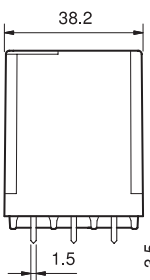
Tipo 62.23 62.23-4300
