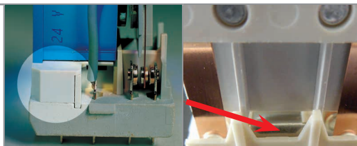
B: Circuito contatti 5, 6 Separatore SELV tra bobina e contatti
