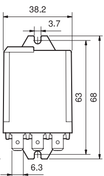
Tipo 62.83 62.83-4300
