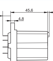
062.10 con relè
