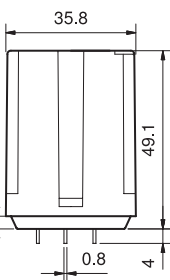
Tipo 62.3x-4300
