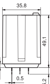
Tipo 62.8x-4300
