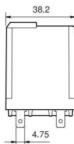
Tipo 62.32 62.32-4300
