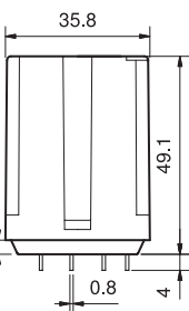
Tipo 62.3x
