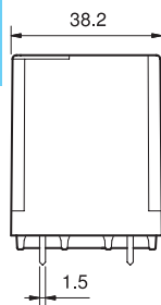
Tipo 62.22 62.22-4300
