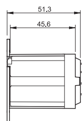
062.05 con relè
