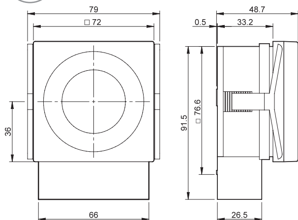
Tipi 12.51/12.81 Morsetti a bussola
