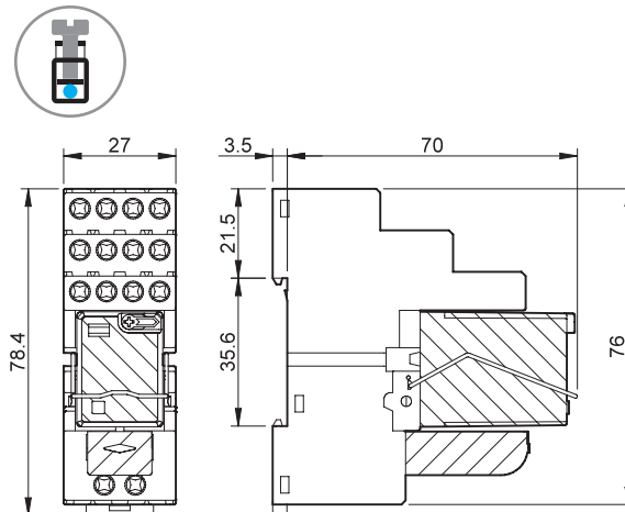
Tipo 58.P4 Morsetti Push-in
