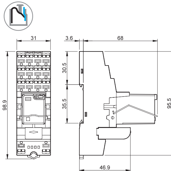
Tipo 58.P4 Morsetti Push-in
