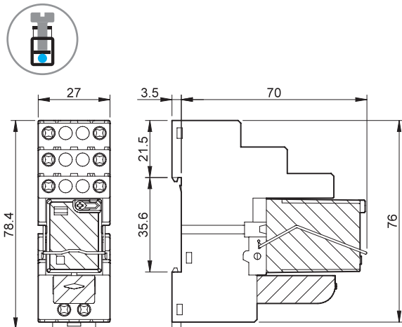
Tipo 58.P3 Morsetti Push-in
