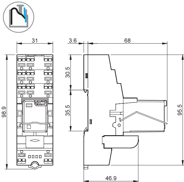
Tipo 58.P3 Morsetti Push-in
